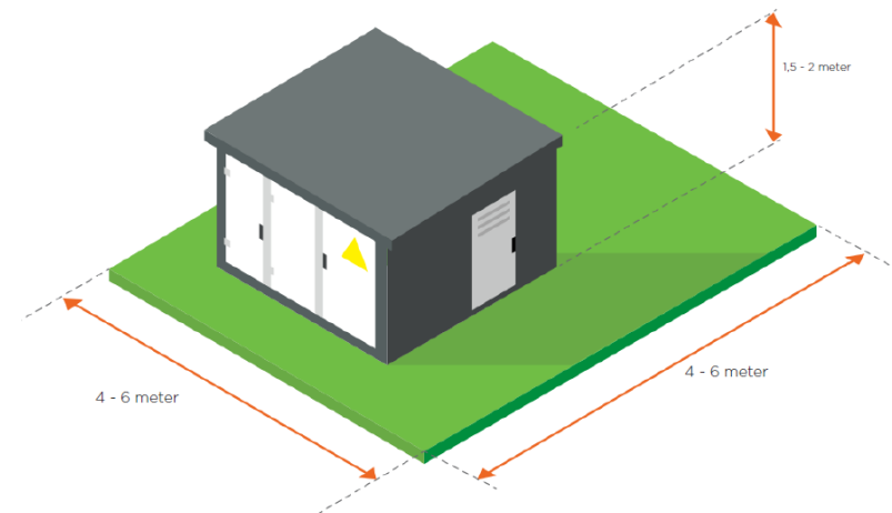
Figuur 8 - Ruimtegebruik middenspanningstation
