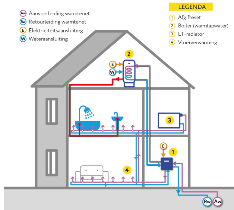
Figuur 3 - Schematische opstelling van een aansluiting op een lagetemperatuurwarmtenet
